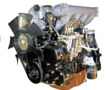
XINCHAI A498BT1
